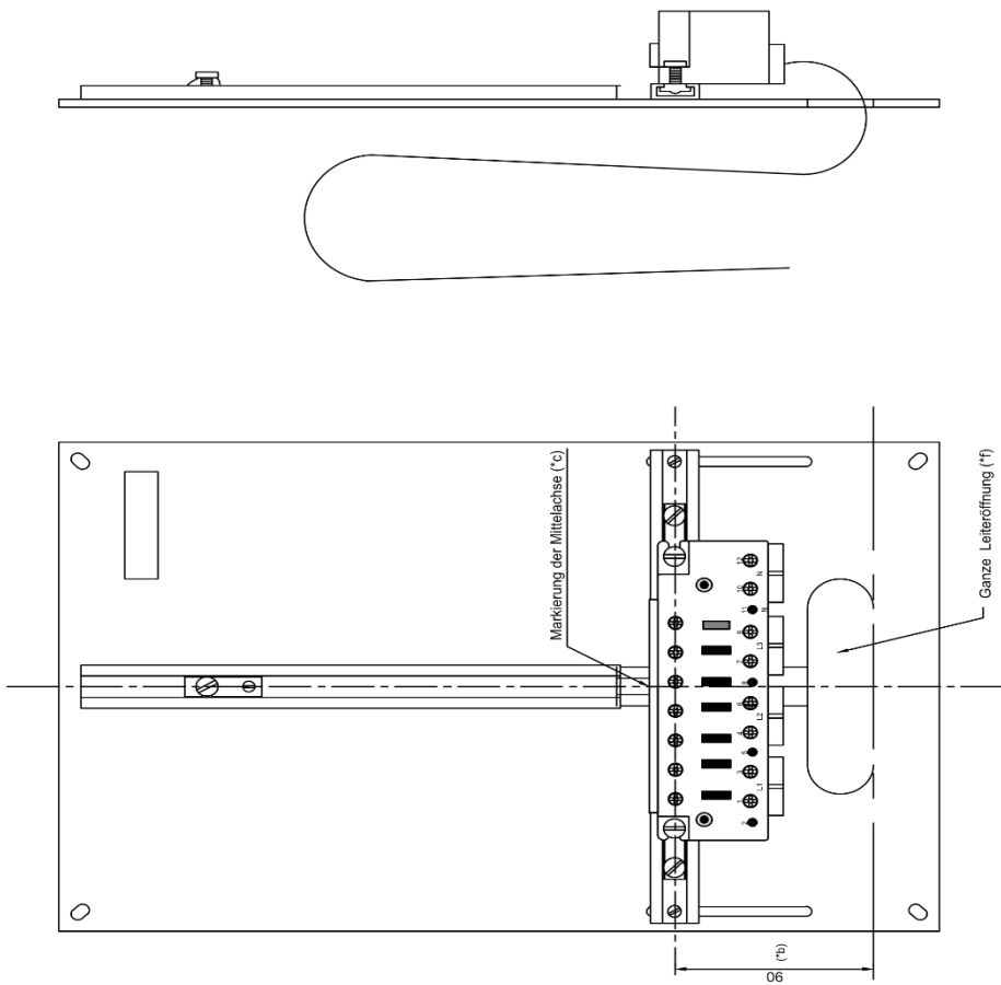
Montagehinweise der 80/100A-Zählersteckklemme (25 mm 2 )
